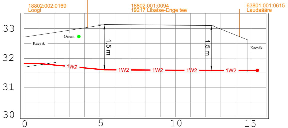
Ristmävli RV-3 Riigitee nr 19207 Libatse-Enge tee teemaal km 4,25 Ø160 13 m 1250N Kinnine läbindamine
